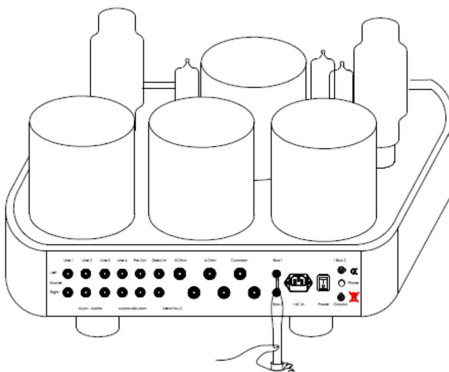
Регулировка напряжения смещения
