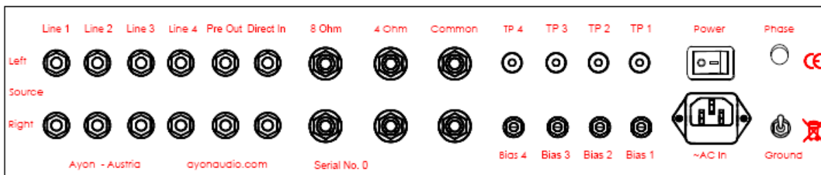
Задняя панель
